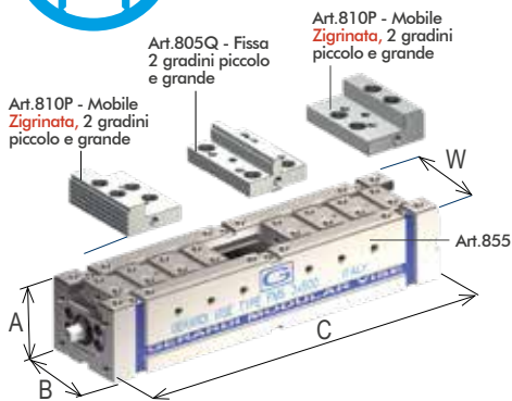
Art.864 Morsa doppia singola autocentrante con ganasce a doppio gradino zigrinate. Disponibile A RICHIESTA con ganasce lisce
