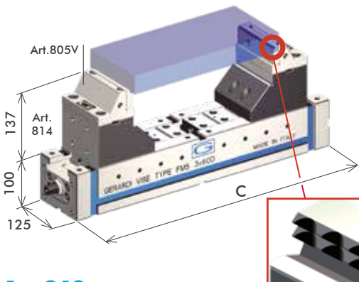
Art.868 Morsa autocentrante (opzione doppia o singola) con ganasce alte. Ideale per centri di lavoro a 5 assi
